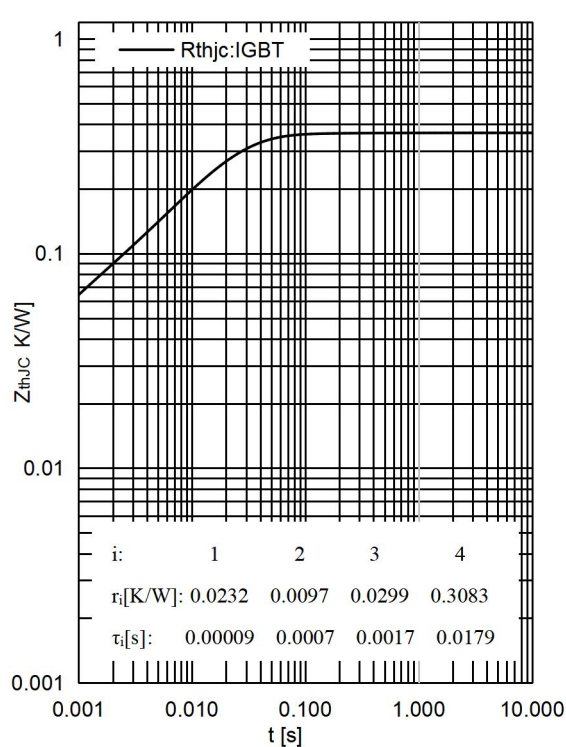
图 6 . IGBT 瞬态热阻抗 Fig 6. IGBT Transient thermal impedance
