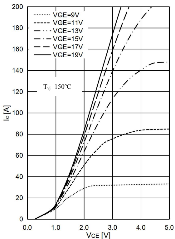
图 2 . IGBT 输出特性
