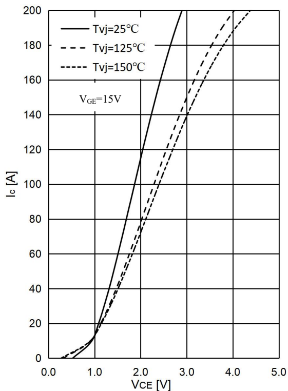
图 1 . IGBT 输出特性
