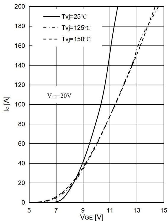
图 3 . IGBT 转移特性
