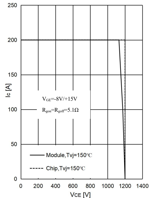
图 7 . IGBT 反偏安全工作区 Fig 7. IGBT RBSOA
