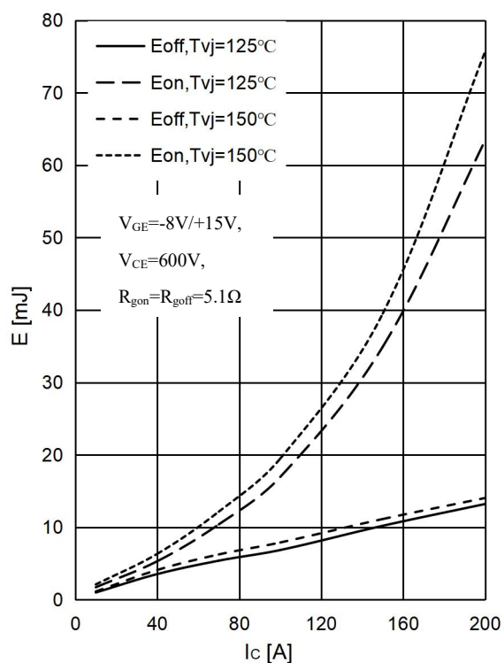
图 4 . IGBT 开关损耗-集电极电流
