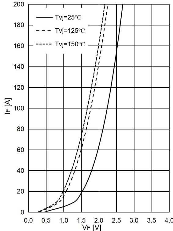
图 8 . 二极管 正向偏压特性 Fig 8. Diode Forward characteristic
