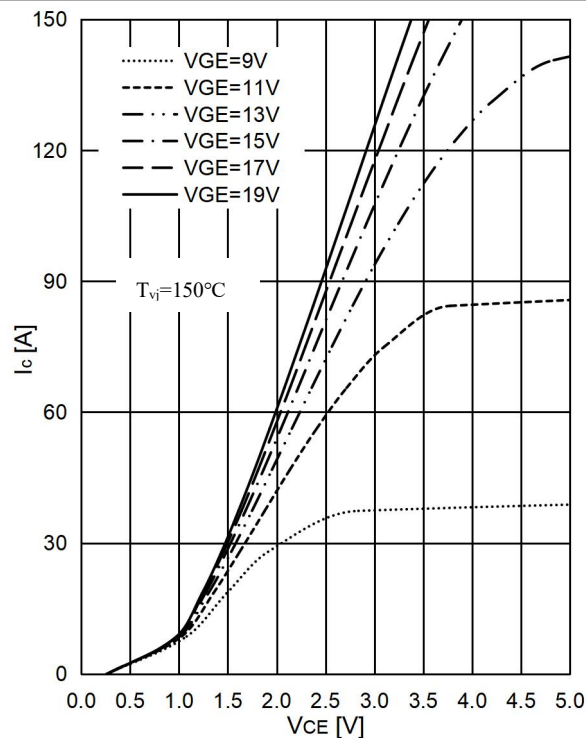
图 2 . IGBT 输出特性,逆变器
