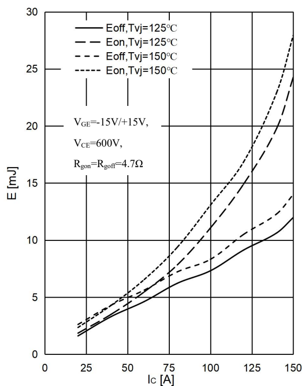
图 4 . IGBT 开关损耗-集电极电流,逆变器
