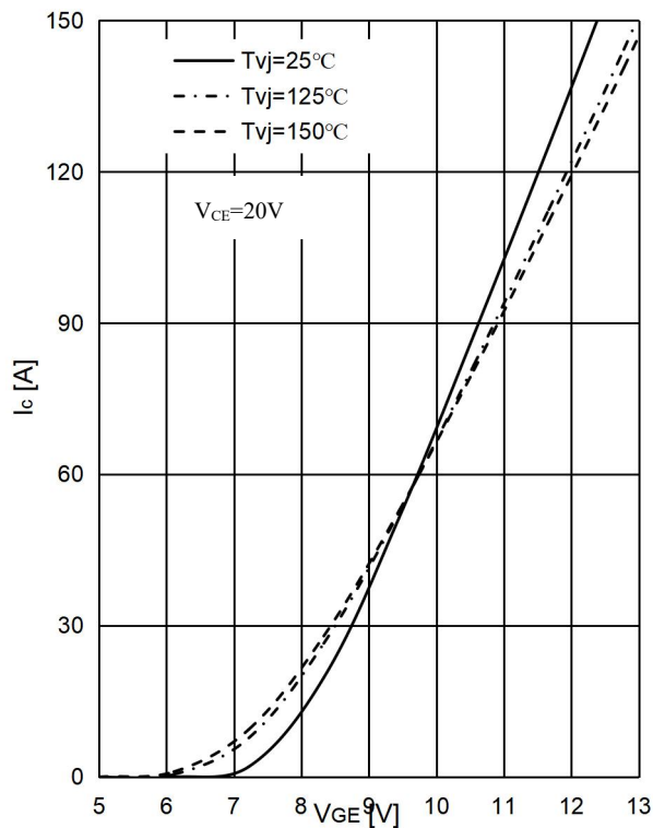
图 3 . IGBT 转移特性,逆变器
