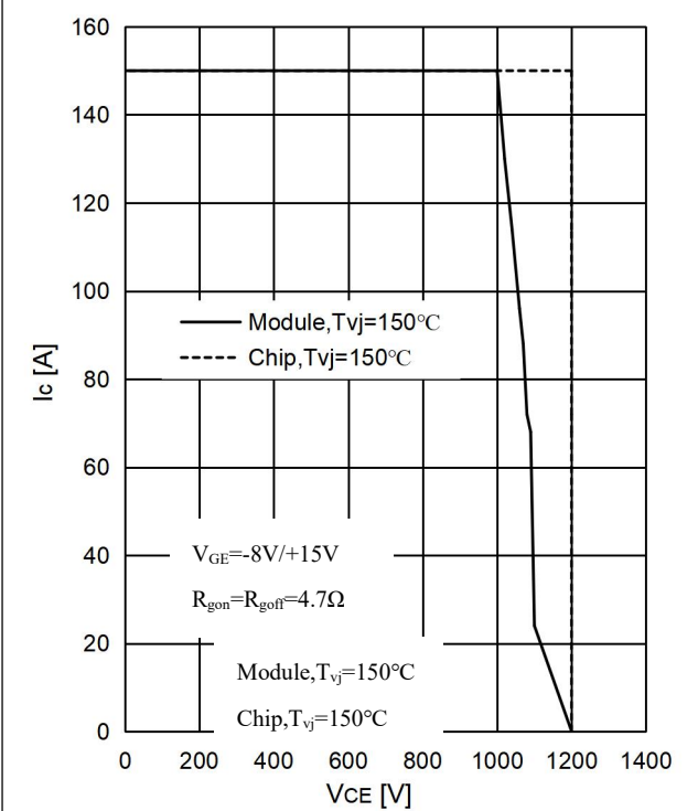
图 7 . IGBT 反偏安全工作区,逆变器 Fig 7. IGBT RBSOA, Inverter
