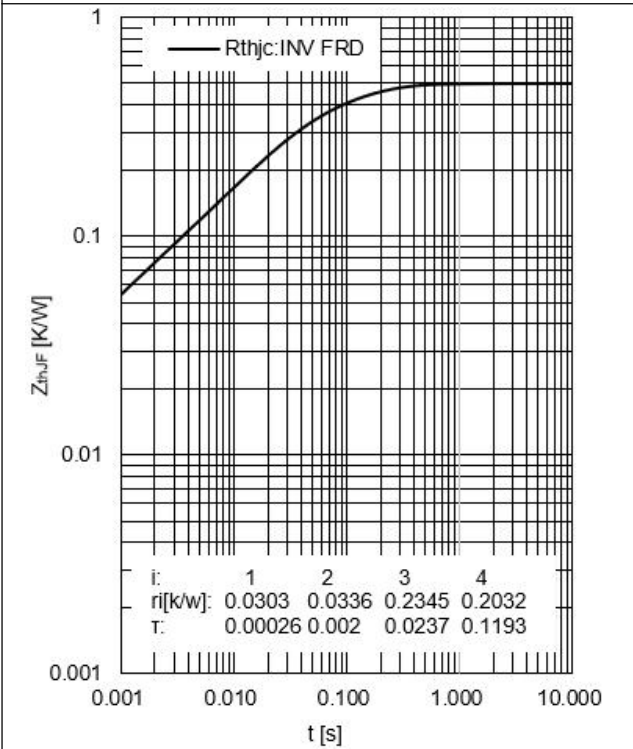
图 11 . 二极管 瞬态热阻抗,逆变器 Fig 11. Diode Transient thermal impedance, Inverter
