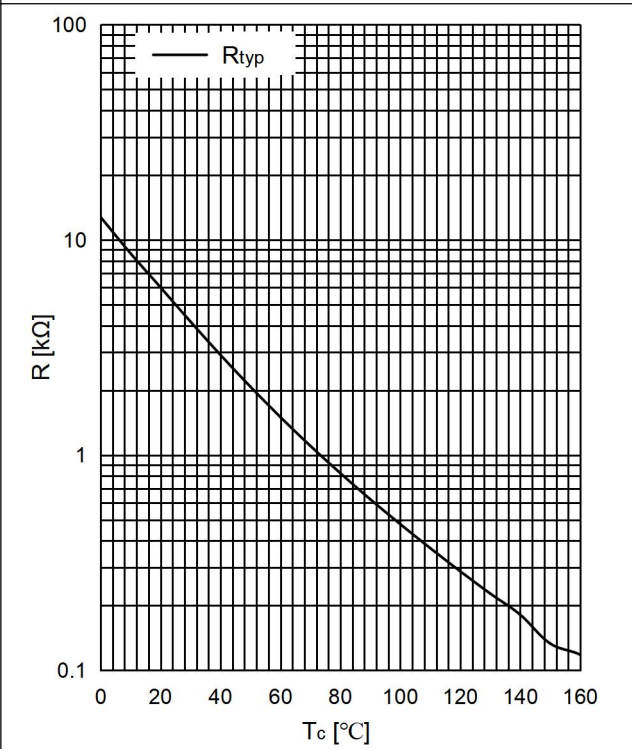
图 12 . 负温度系数热敏电阻 温度特性 Fig 12. NTC-Thermistor-temperature characteristic
