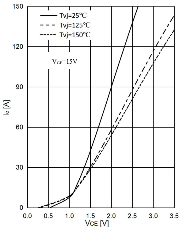
图 1 . IGBT 输出特性,逆变器
