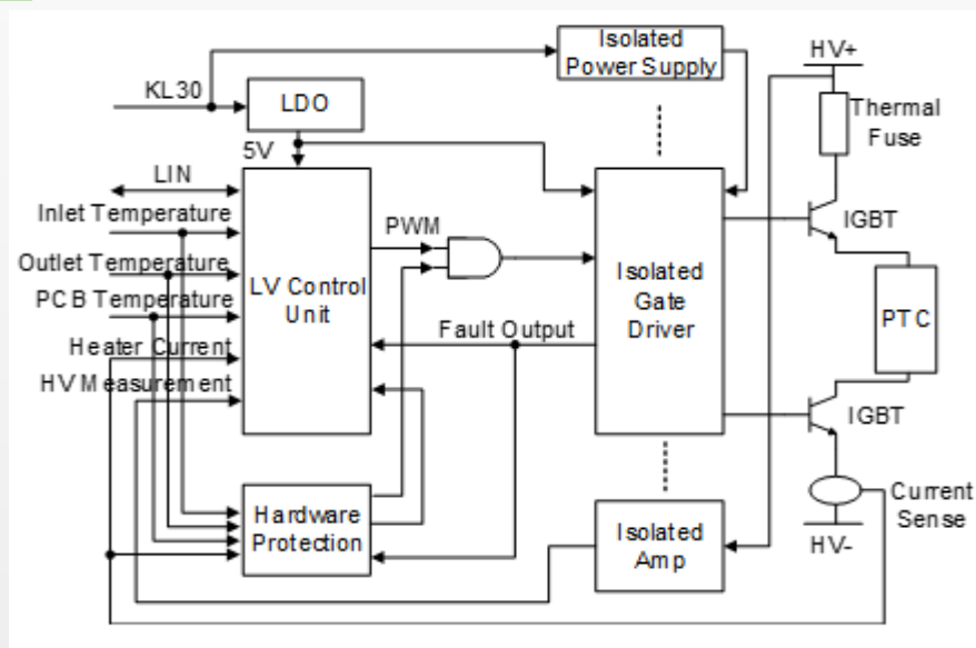
PTC 典型应用电路
