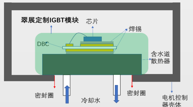
用翠展集成散热水道 IGBT 模块的电机控制器
