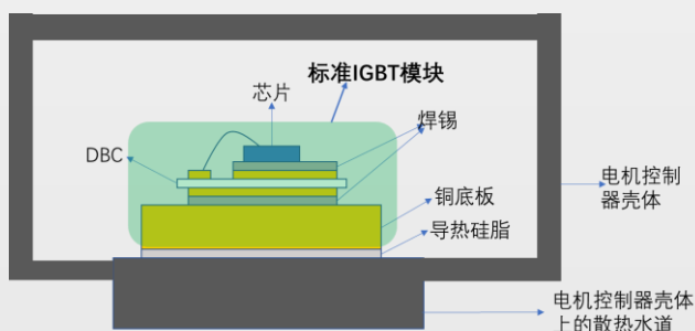
用常规 IGBT 模块的电机控制器
