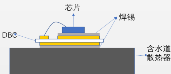
翠展集成散热水道的 IGBT 模块
