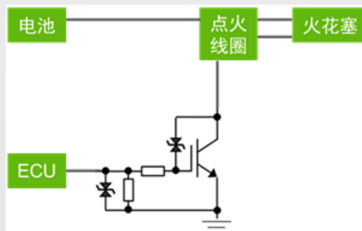
点火 IGBT 典型应用
